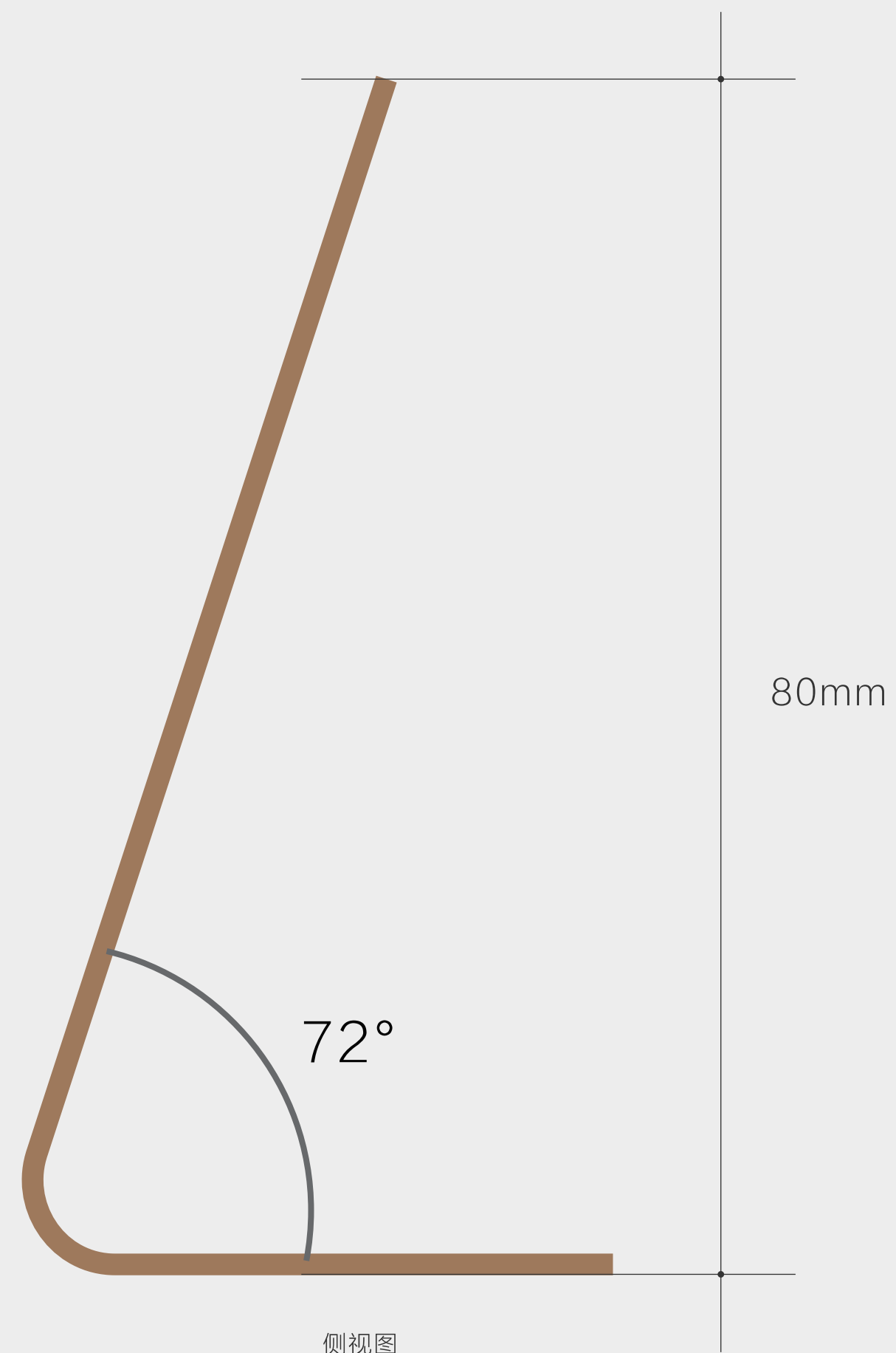
侧视图
